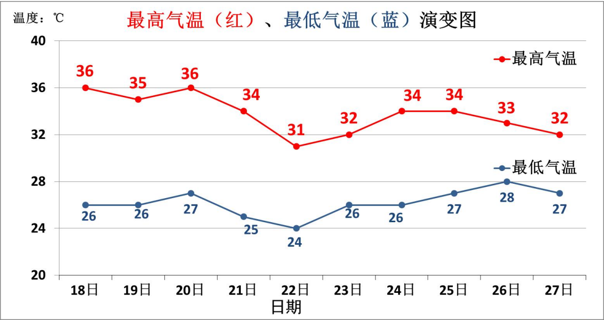
图 17 月 18～27 日南阳市最高气温、最低气温演变图
